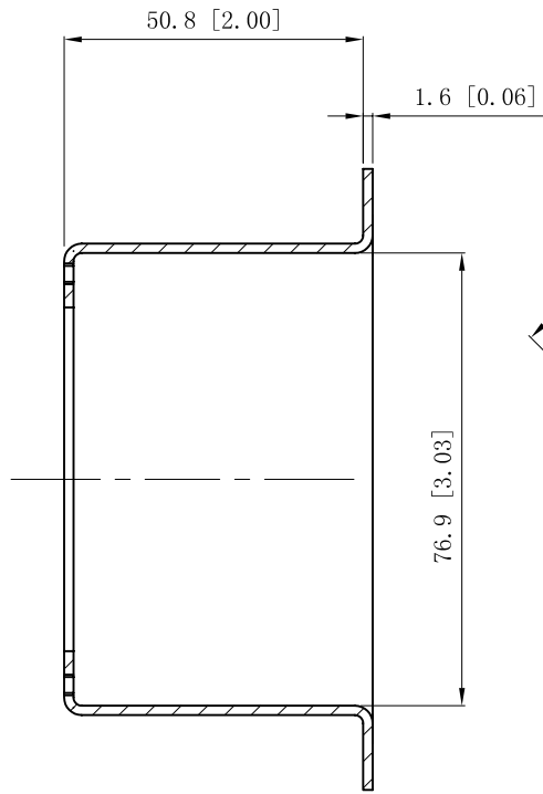
VIEW A-A
