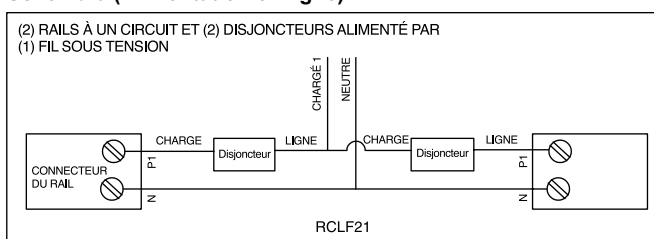
Schéma 4 (Alimentation en ligne)
