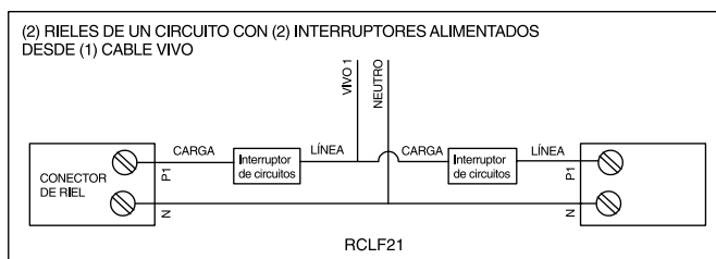
Diagrama 4 (Alimentación en línea)
