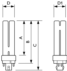
PL-C 18W/835/4P/ALTO 10PK
