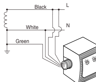
Single-phase 2-wire / Una fase, 2 hilos / Monophasée, 2 fils (+ GND) 120 V~
