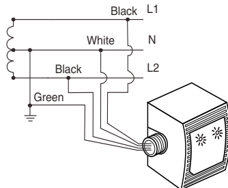
Single-phase 3-wire / Una fase, 3 hilos / Monophasée, 3 fils (+ GND) 120/240 V~
