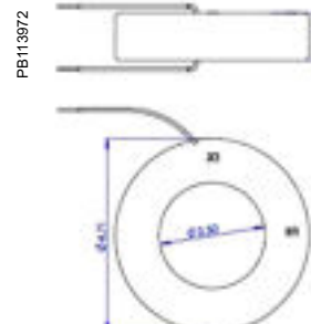
400 A CT dimensions
