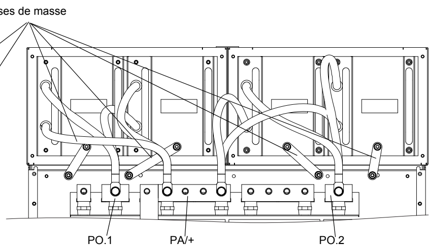
Exemple 4 : ATV71HC40N4 ... C50N4
