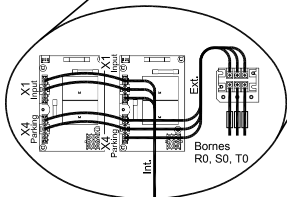
Câblage sortie d'usine : ventilateurs alimentés en interne par R/L1, S/L2, T/L3
