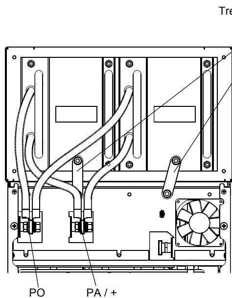
Exemple 2 : ATV71HC16N4 ... C28N4
