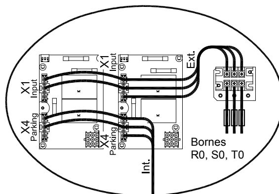
Modification pour ventilateurs alimentés en externe par R0, S0, T0
