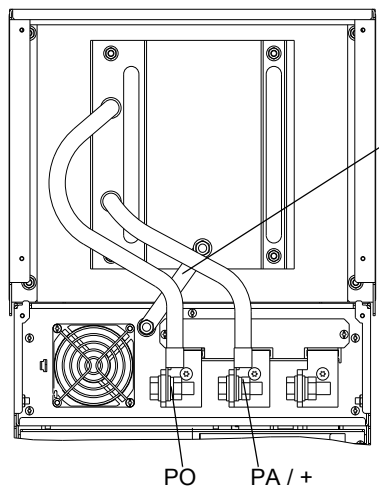
Exemple 1 : ATV71HD55M3X ... D75M3X, ATV71HD90N4 ... C13N4
