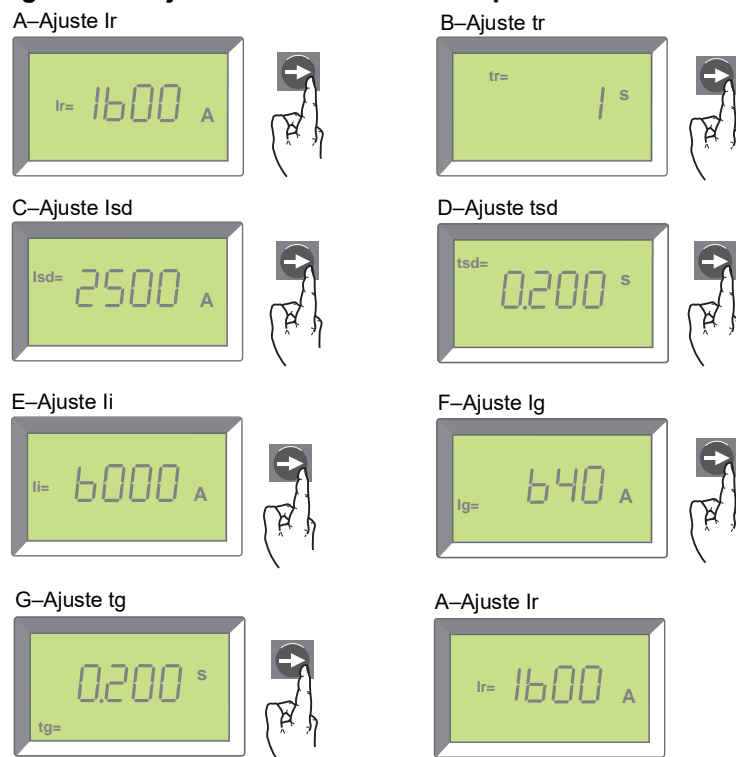
Figura 21 – Ajustes de la unidad de disparo
