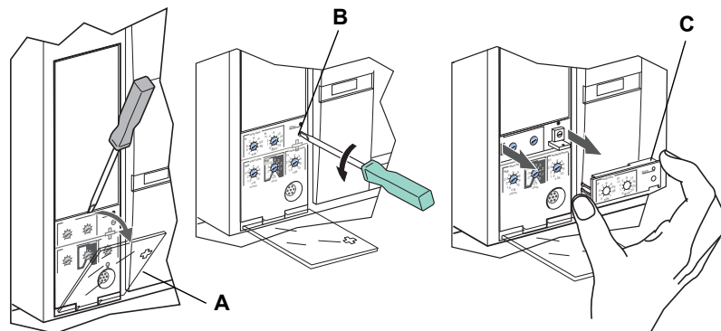
Figura 49 – Extracción del calibrador ajustable
