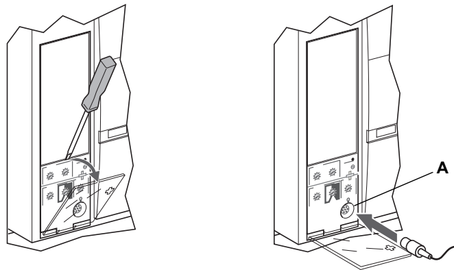
Figura 38 – Verificación del funcionamiento de la unidad de disparo
