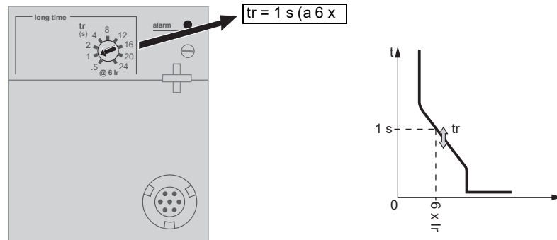
Figura 28 – Ajuste del retardo de tiempo
