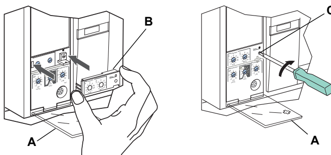
Figure 47: Installation de la fiche de valeur nominale réglable
