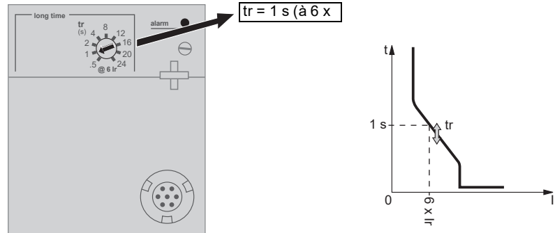
Figure 26 – Régler la temporisation
