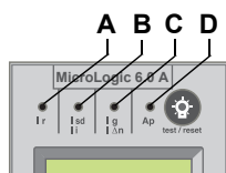
Figure 12 – Voyants de déclenchement
