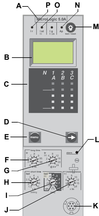
Figura 4 – Unidad de disparo 5.0A
