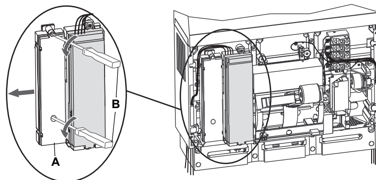
Figura 51 – Desplazamiento del módulo de aguante
