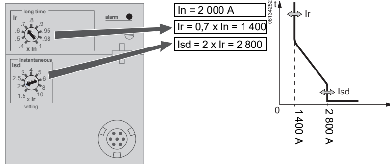
Figura 25 – Ajuste de los niveles de activación
