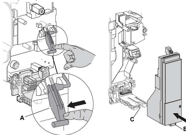
Figura 46 – Instalación de la unidad de disparo
