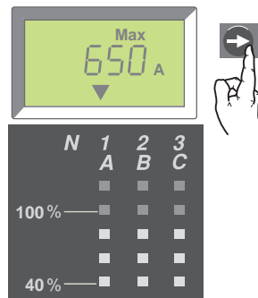
Figura 19 – Corrientes máximas
