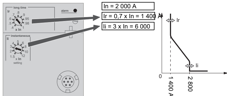
Figure 27 – Régler les niveaux d'enclenchement
