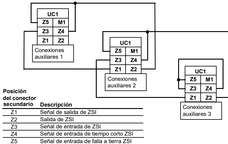
Figura 34 – Ejemplo de cableado de ZSI
