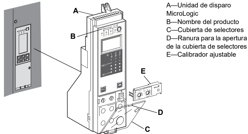
Figura 1 – Unidad de disparo MicroLogic
