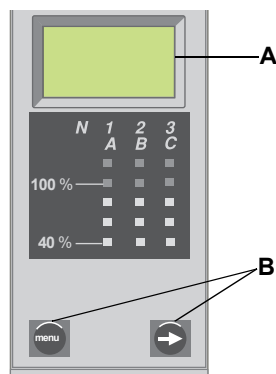
Figure 13 – Ampèremètre
