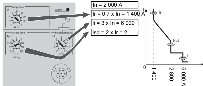
Figure 29 – Régler les niveaux d'enclenchement
