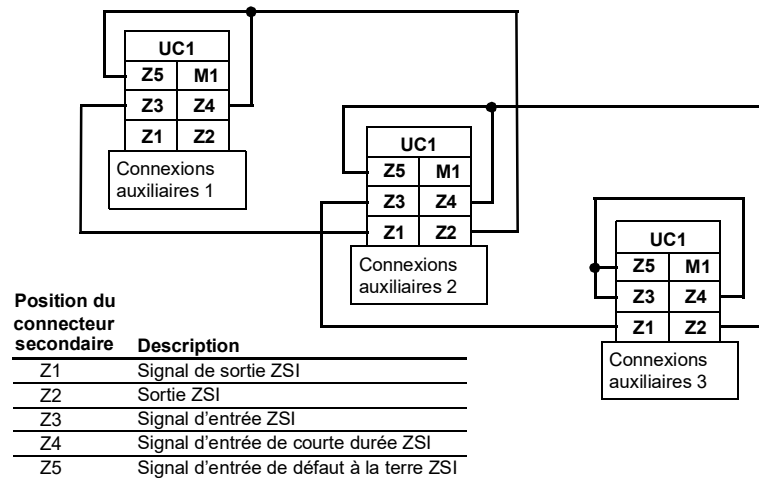
Figure 34 – Exemple de câblage ZSI
