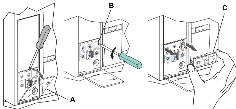
Figura 42 – Desmontaje del calibrador ajustable
