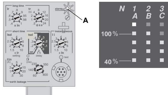
Figura 11 – Luz indicadora de sobrecarga
