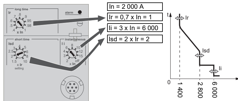
Figura 29 – Ajuste de los niveles de activación
