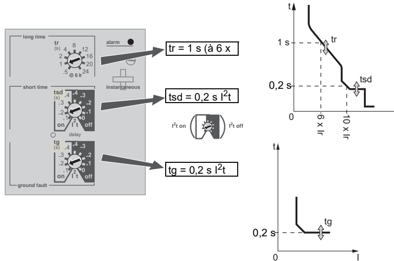
Figure 32 – Régler les temporisations
