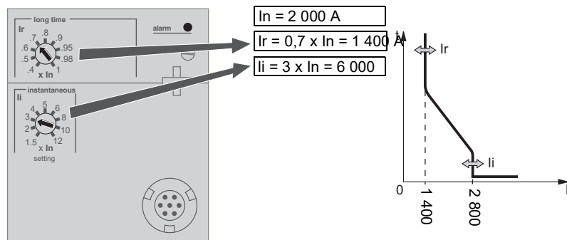
Figura 27 – Ajuste de los niveles de activación
