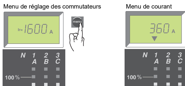
Figure 22 – Revenir au menu de courant
