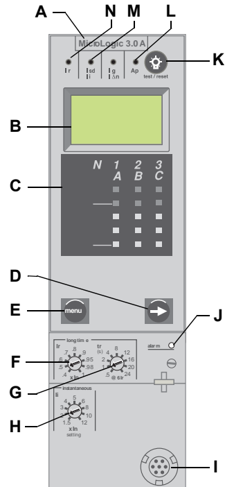
Figure 3 – Déclencheur 3.0A
