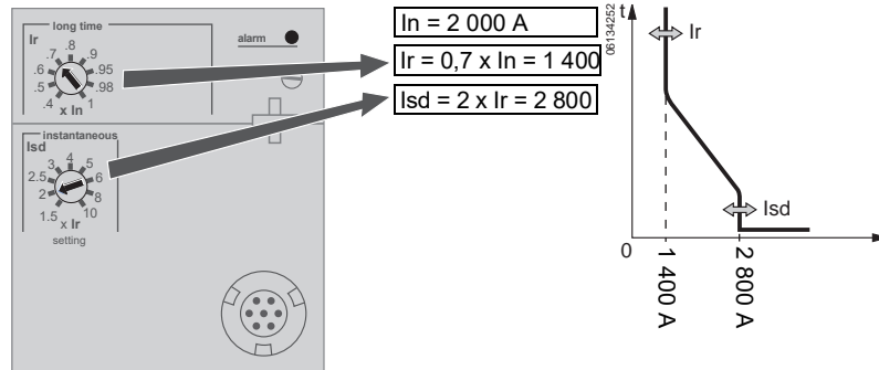
Figure 25 – Régler les niveaux d'enclenchement
