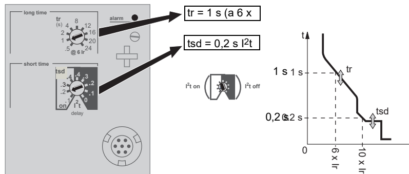
Figura 30 – Ajuste del retardo de tiempo
