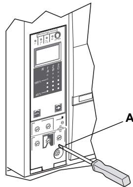
Figura 39 – Prueba de las funciones de disparo por falla a tierra del equipo
