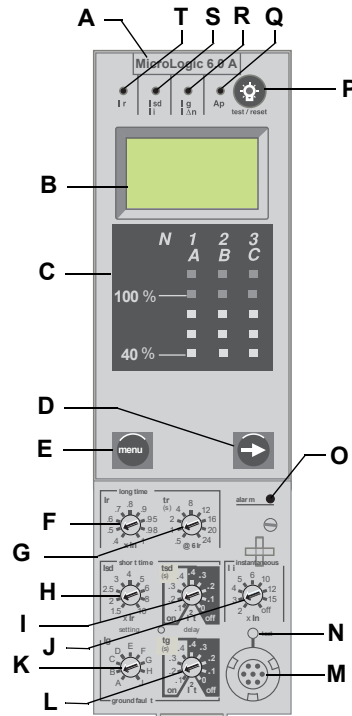
Figura 5 – Unidad de disparo 6.0A
