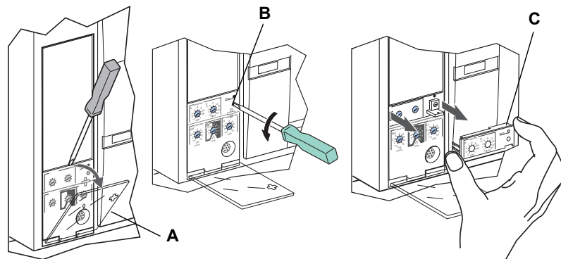
Figure 48 – Enlever la fiche de valeur nominale réglable
