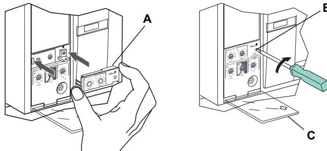
Figure 49 – Installer la nouvelle fiche de valeur nominale réglable
