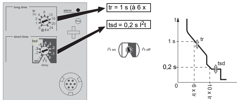
Figure 30 – Régler les temporisations
