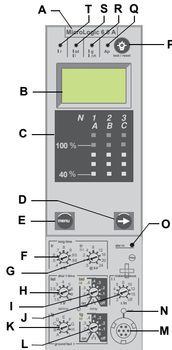
Figure 5 – Déclencheur 6.0A
