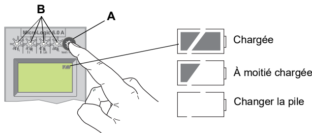
Figure 40 – Vérification de l'état du déclencheur
