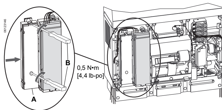
Figure 53 – Replacer le module de tenue
