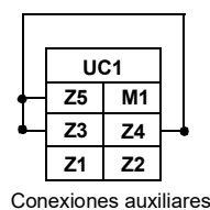
Figura 33 – Terminales en puente
