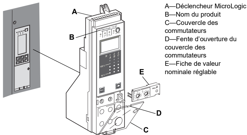
Figure 1 – Déclencheur MicroLogic
