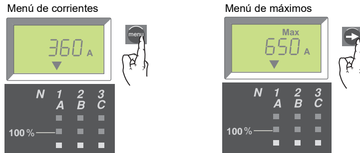
Figura 18 – Acceso al menú de máximos
