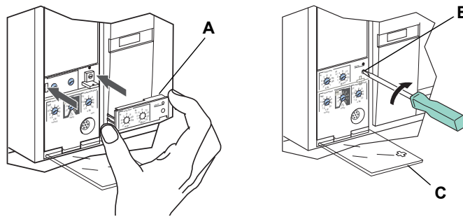
Figura 50 – Instalación del nuevo calibrador ajustable
