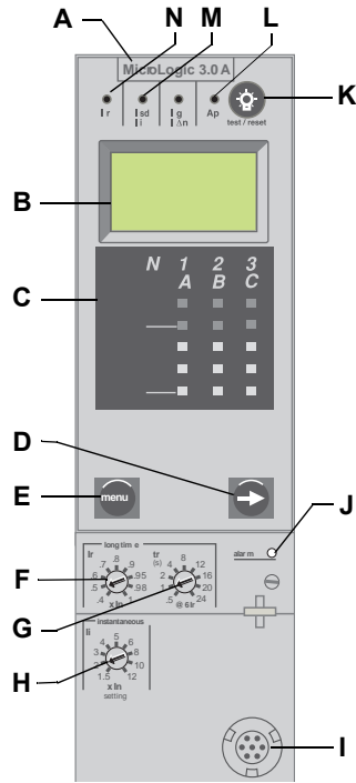
Figura 3 – Unidad de disparo 3.0A
