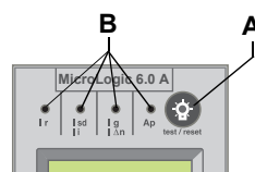
Figura 45 – Luces indicadoras
