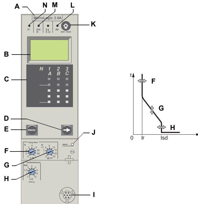
Figura 2 – Unidad de disparo 2.0A
