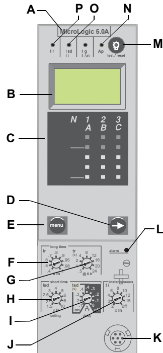
Figure 4 – Déclencheur 5.0A
