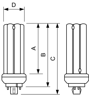
PL-T 26W/827/A/4P/ALTO
