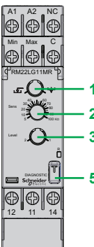
RM22LG11MR
