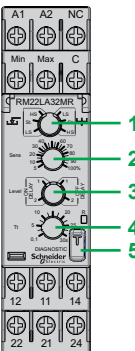
RM22LA32MR
