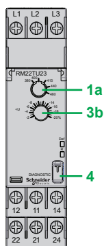
RM22TU
