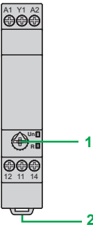
RM17JC00MW
