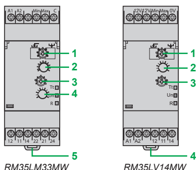
RM35LM33MW
