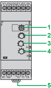
RM35S0MW
