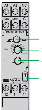
RM22LG11MT
