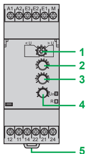
RM35 UA11MW/UA12MW/UA13MW
