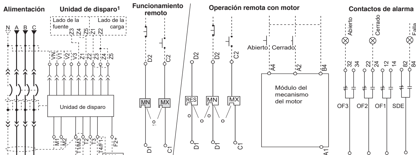
FIG. 4 : Diagramas del cableado de control de los accesorios (Espanol)
