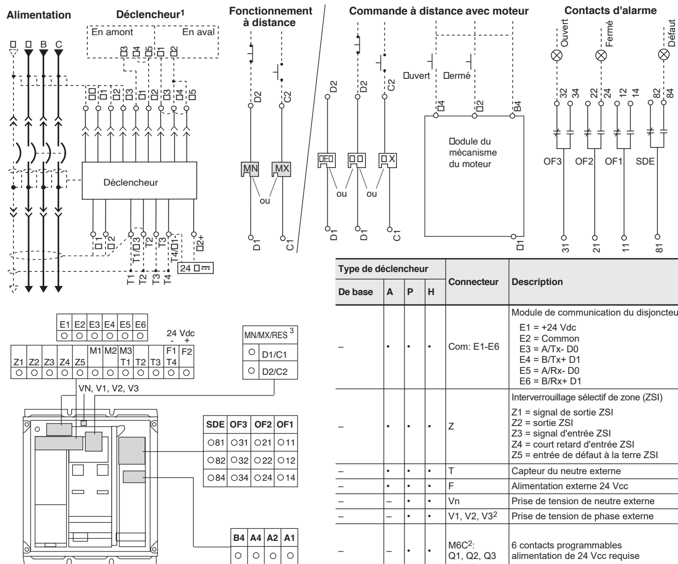
FIG. 5 : Schémas de câblage de commande des accessoires (Français)
