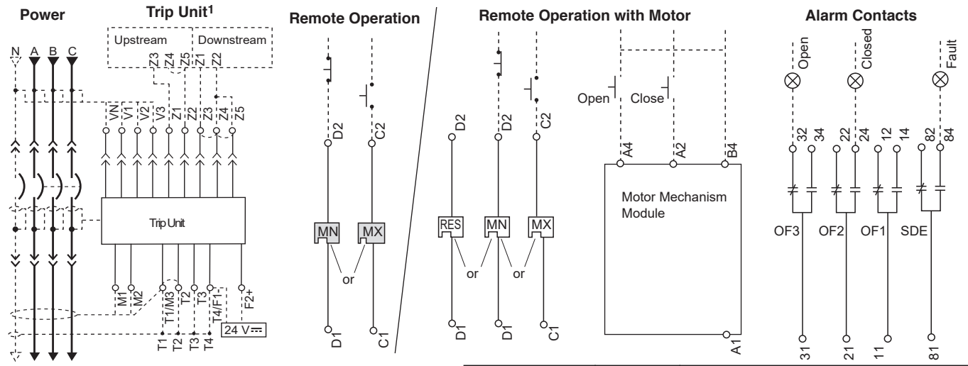
FIG. 3 : Accessory Control Wiring Diagrams (English)
